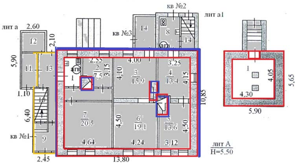
ПЛАН 1 ЭТАЖ
