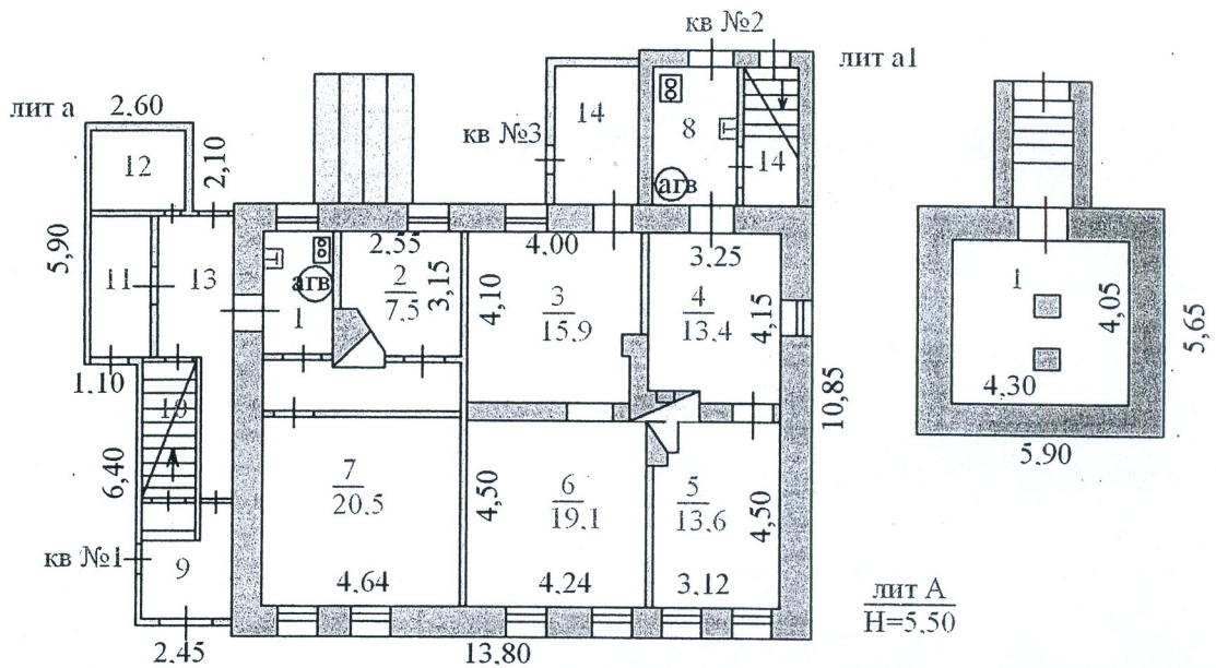
ПЛАН 1 ЭТАЖ
