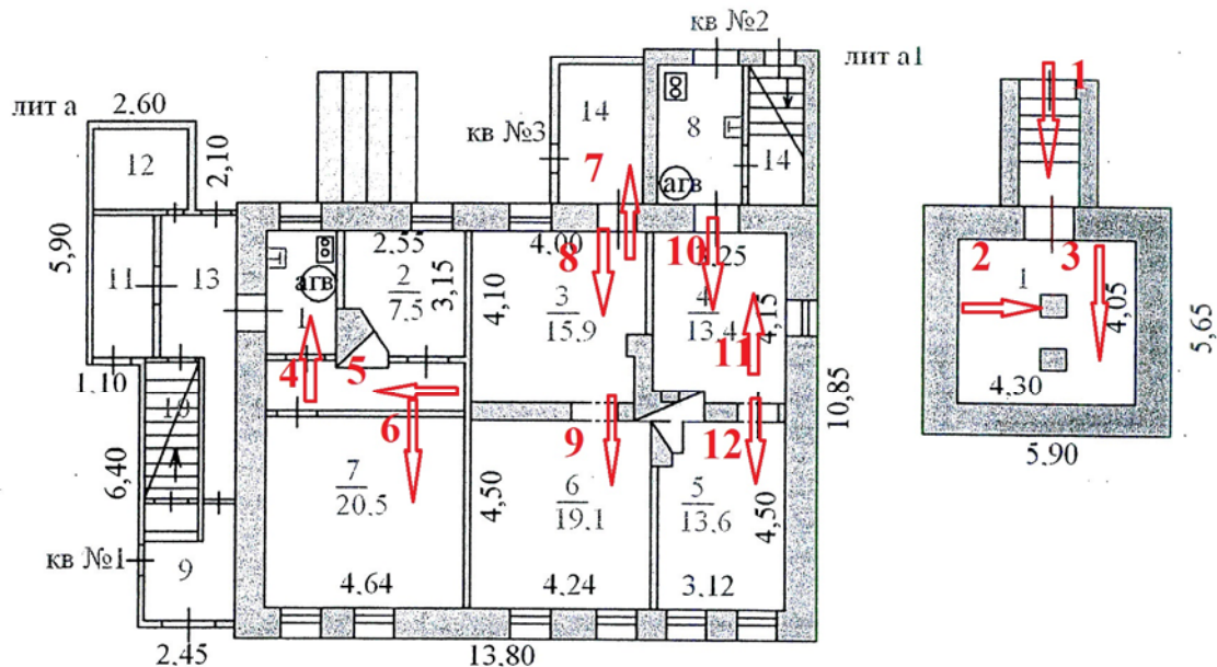
ПЛАН 1 ЭТАЖ
